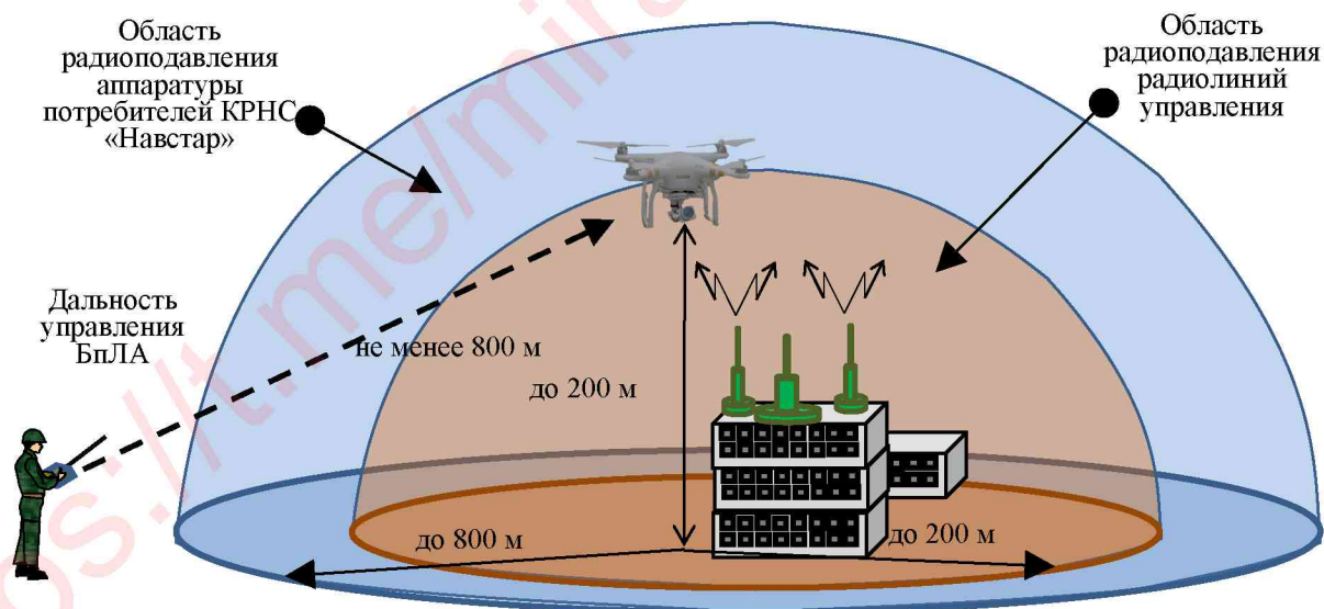
Рис. 13. Вариант применения станции помех РП-377УВМ1Л «Лесочек», при РЭП радиолиний управления и аппаратуры потребителя КРНС БПЛА
