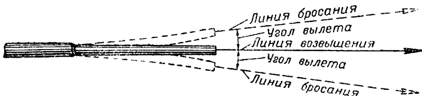
Рис. 50. Колебания ствола во время выстрела.
