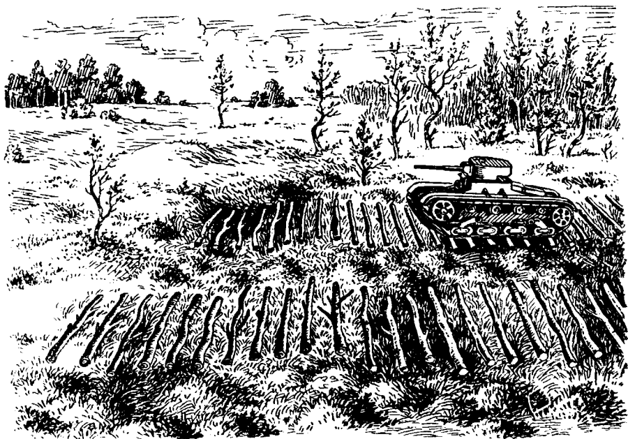
Рис. 106. Жердевая дорожка.
