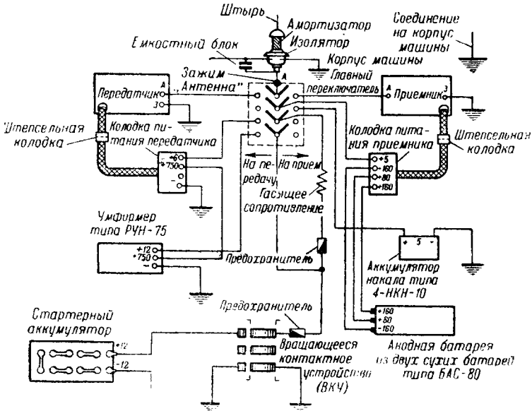
Рис. 155. Схема монтажа танковой радиостанции.
