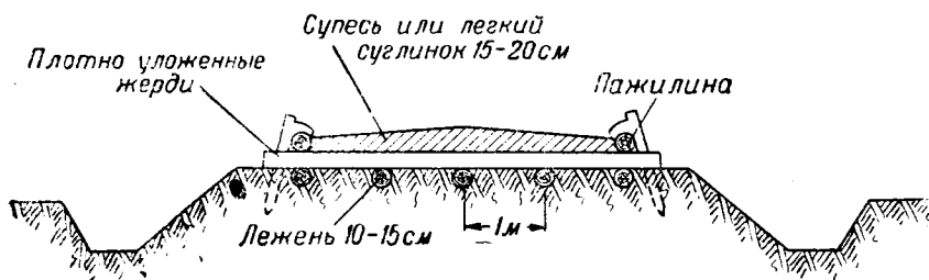
Рис. 109. Жердевой настил.
