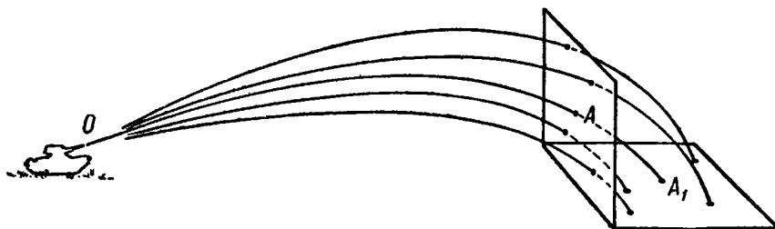
Рис. 61. Рассеивание выстрелов при стрельбе с места ( ОАА_1 — средняя траектория А и А_1 — средние точки попадания).
