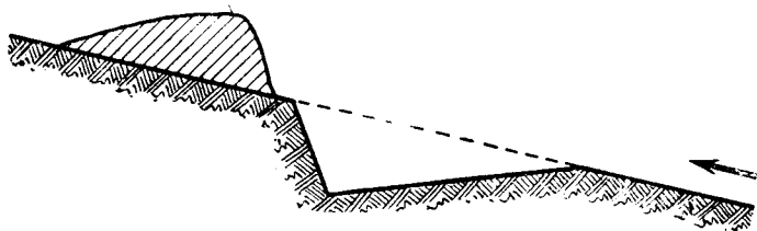
Рис. 129. Эскарп.
