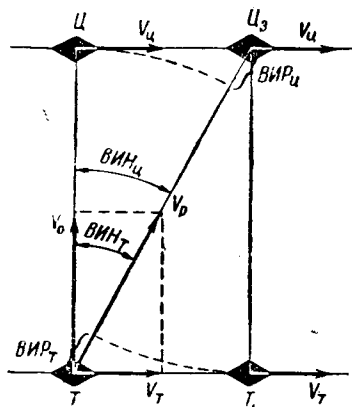
Рис. 91. Изменение расстояния и направления стрельбы при стрельбе с хода по движущейся цели (движение равноименными бортами).
