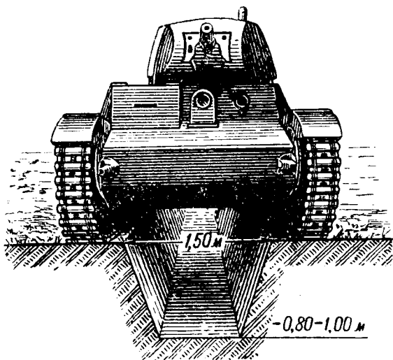
Рис. 140. Укрытие (щель) для экипажа танка.
