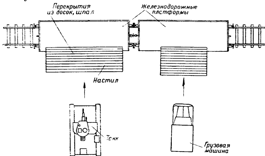
Рис. 180. Боковые погрузочные мостки.
