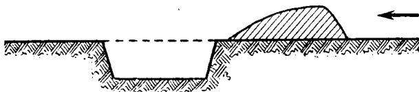
Рис. 127. Ров с обратным бруствером.
