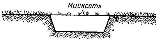
Рис. 125. Ров без бруствера.
