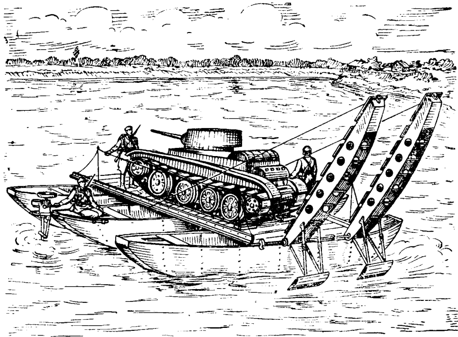
Рис. 113. Паром из понтонов ИЭП.
